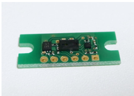
センサ基板 (部品ハンダ付け済)
