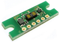
ST マイクロエレクトロニクス VL53L1X 搭載
