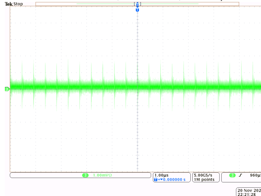
出力 1.2V 時の出力ノイズ特性 (VIN=12V, VOUT=1.2V, LOAD=1A, S-CONF=VIN, BW=1GHz, Z=50Ω)
