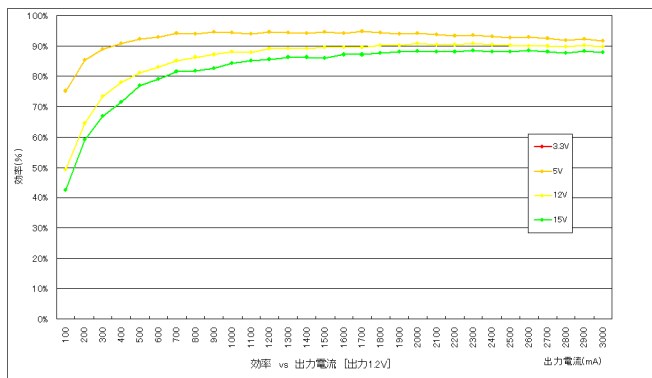
出力 1.2V 時の負荷電流・効率特性 (S-CONF=VIN)
