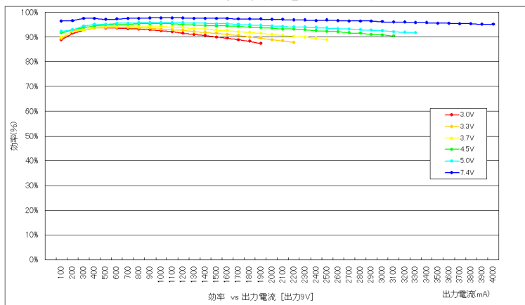
▼出力 9V 時の負荷電流・効率特性
