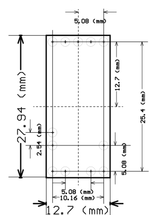
■寸法図 (穴径はすべて 1.0mm です)
