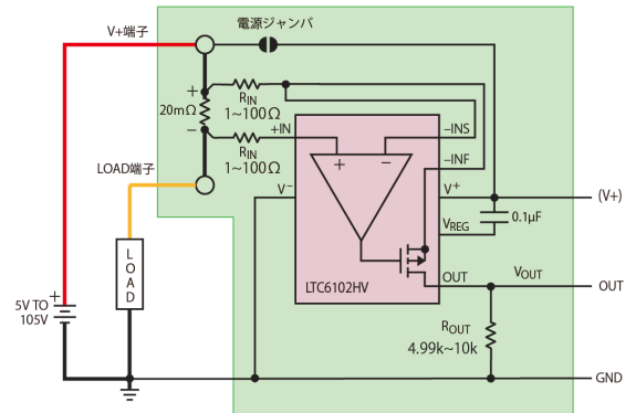
全体のブロック図 (緑色内がこのモジュールの回路です)
