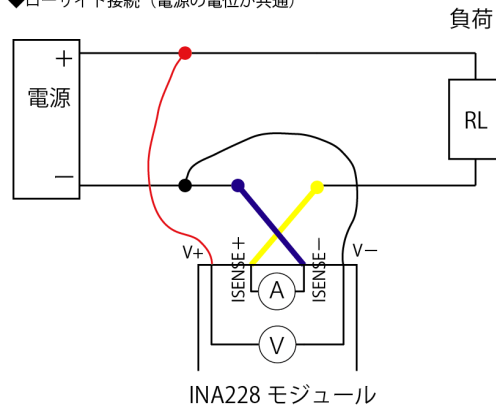
◆ローサイド接続 (電源の電位が共通)
