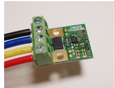
●標準組み立て例
