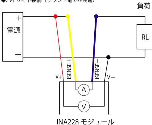
◆ハイサイド接続 (グラウンド電位が共通)
